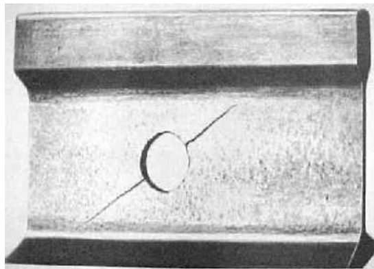
FIG. 45 : 135 OR 235 - WEB , CRACKS AT HOLE
